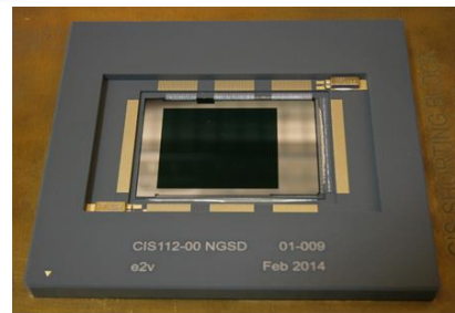
NGSD CIS112 880X840
