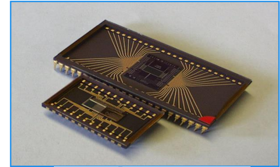
EM CCD60 128X128
