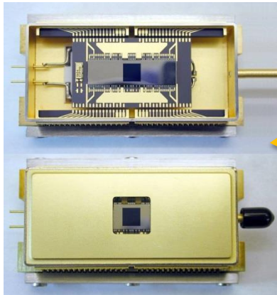
EM CCD220 240X240
